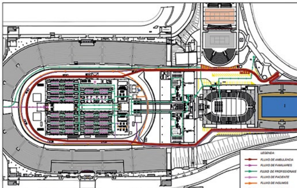
FIGURA 2. Hospital Municipal do Pacaembu: A- planta baixa; B – fotografia externa
